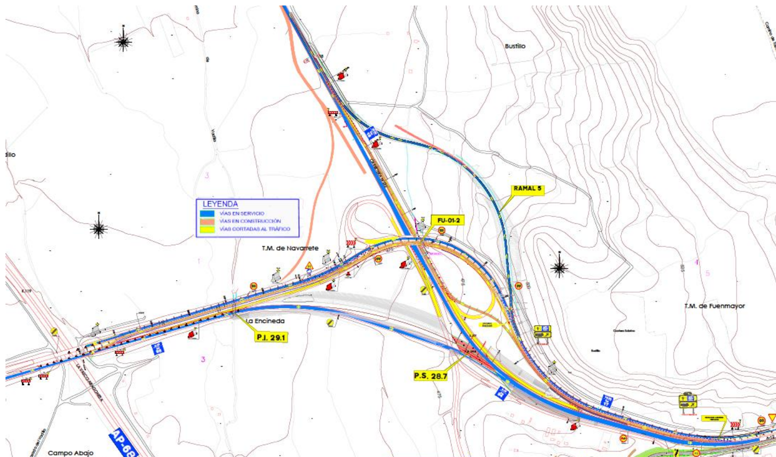
Traslado de tráfico de la LO-20 dirección Vitoria/Fuenmayor al ramal 5
