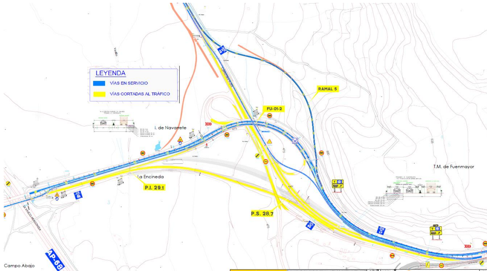
Traslado del tráfico de la A-12 dirección Logroño a calzada A-12 dirección Burgos y mediana acondicionada. Traslado tráfico N-232 dirección Logroño a vial provisional.
